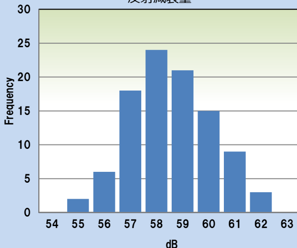
反射減衰量
